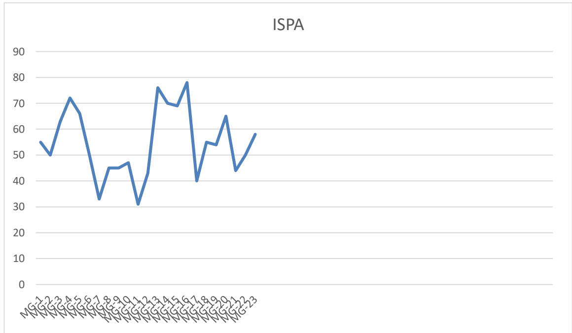
Grafik 6. Tren Penemuan ISPA diKecamatan Belakang Padang Minggu ke-23 Tahun 2026
