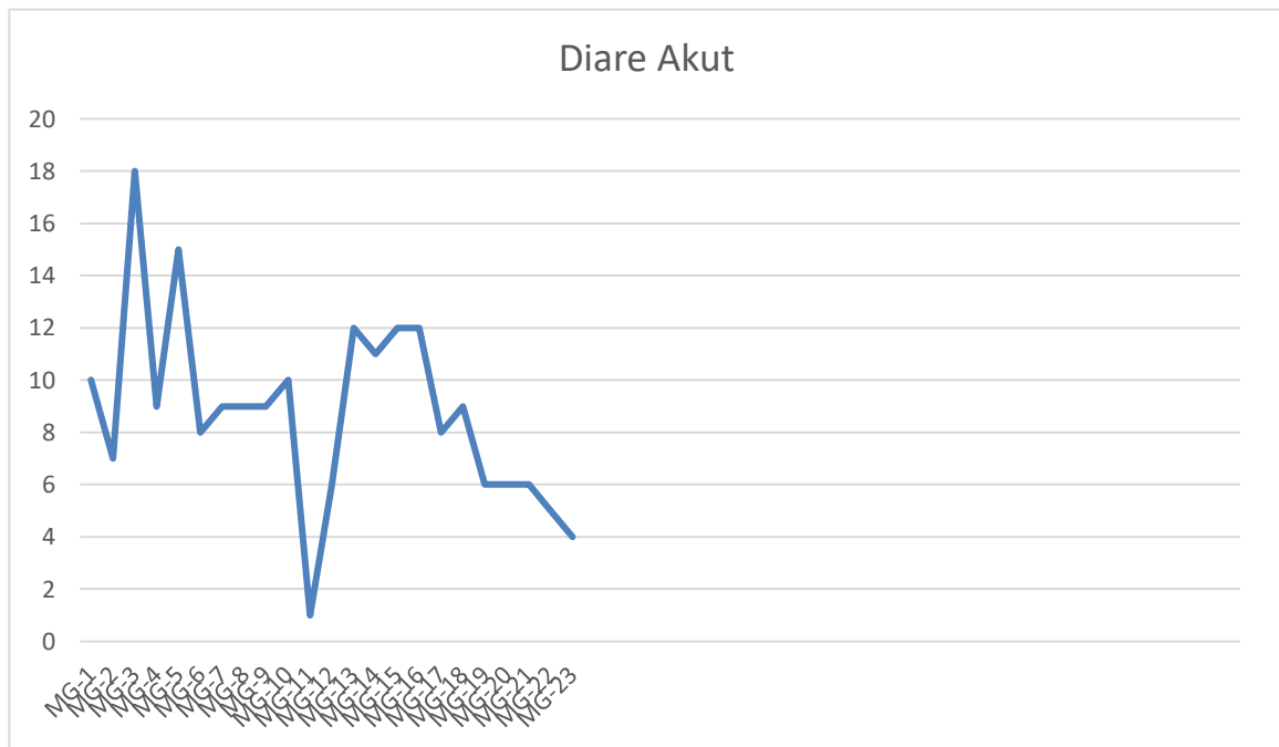
Grafik 1. Tren Penemuan Diare Akut di Kecamatan Belakang Padang Minggu 1-23 Tahun 2026
