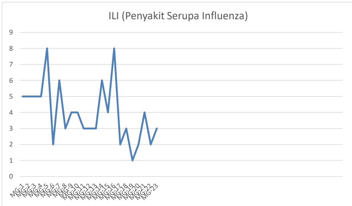
Grafik 5. Tren Penemuan ILI ( Penyakit Serupa Influenza) di Kecamatan Belakang Padang Minggu 1-23 Tahun 2026
