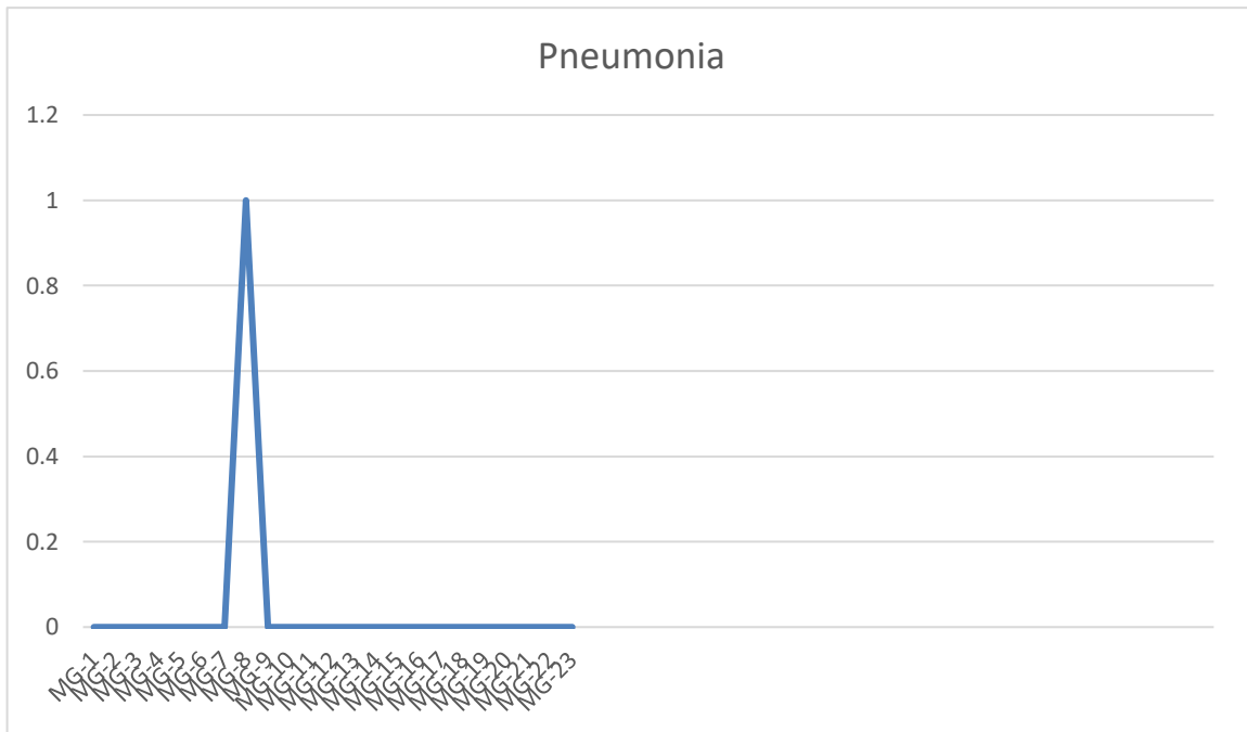
Grafik 2. Tren Penemuan Pneumonia diKecamatan Belakang Padang Minggu 1-23 Tahun 2025
