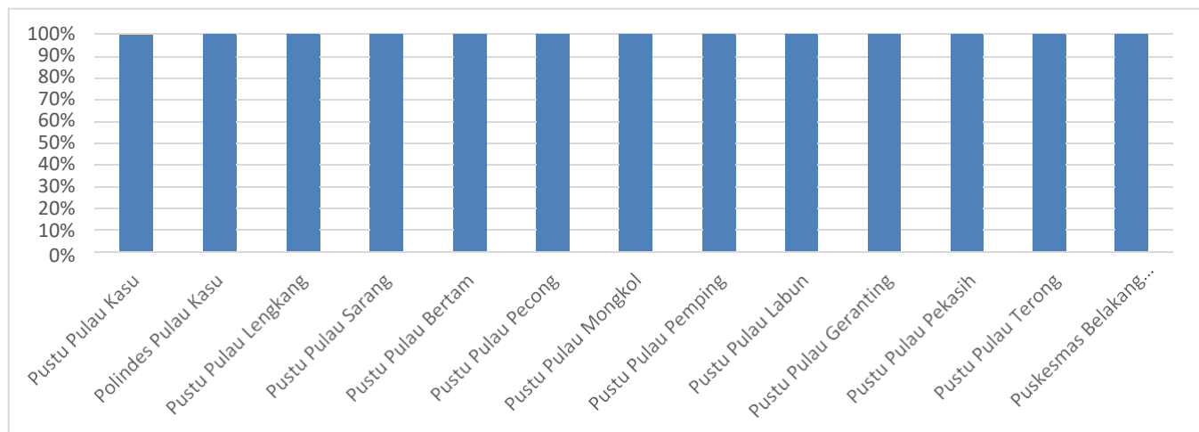
Grafik 1. Kelengkapan Laporan SKDR di Kecamatan Belakang Padang Kota Batam Kepulauan Riau Minggu ke-23 tahun 2026
