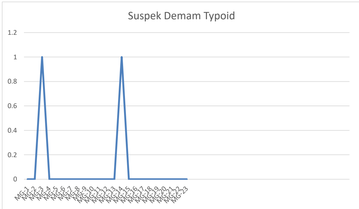
Grafik 3. Tren Penemuan Suspek Demam Typoid di Kecamatan Belakang Padang Minggu 1-23 Tahun 2026
