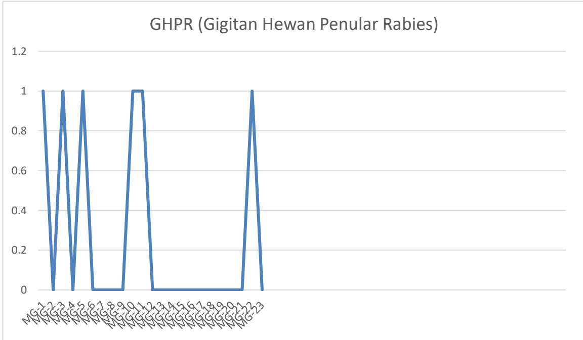
Grafik 4. Tren Penemuan GHPR di Kecamatan Belakang Padang Minggu 1-23 Tahun 2026
