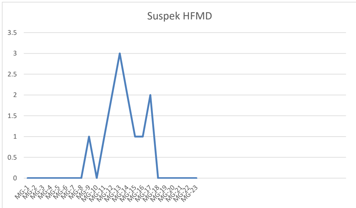
Grafik 6. Tren Penemuan Suspek HFMD diKecamatan Belakang Padang Minggu 1-23 Tahun 2025
