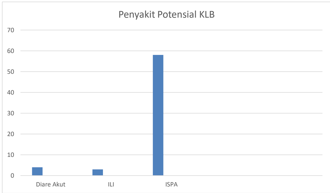
Grafik 1. Penyakit potensial KLB di Kecamatan Belakang Padang Kota Batam Kepulauan Riau Minggu ke-23 Tahun 2026
