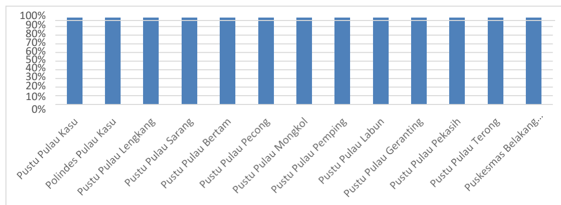
Grafik 2. Ketepatan Laporan SKDR di Kecamatan Belakang Padang Kota Batam Kepulauan Riau Minggu ke-23 tahun 2026
